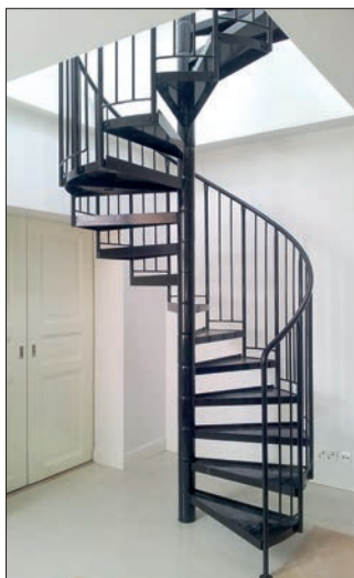
Vakiopinnakaide koostuu \varnothing 26,9 mm kaidetolpista ja niiden väliin tulevasta \varnothing 12 mm teräspinnasta. Tämän portaatan askelmissa on syvennys lattiamatolle.
